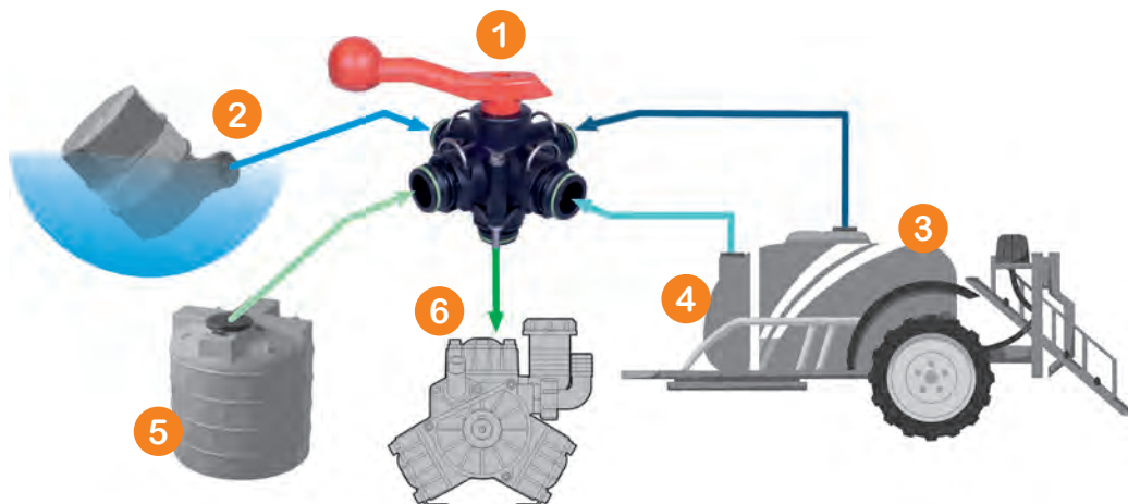
ESEMPIO DI COLLEGAMENTO VALVOLE KH - CONNECTION EXAMPLE KH VALVES EJEMPLO DE CONEXIÓN VÁLVULAS KH
