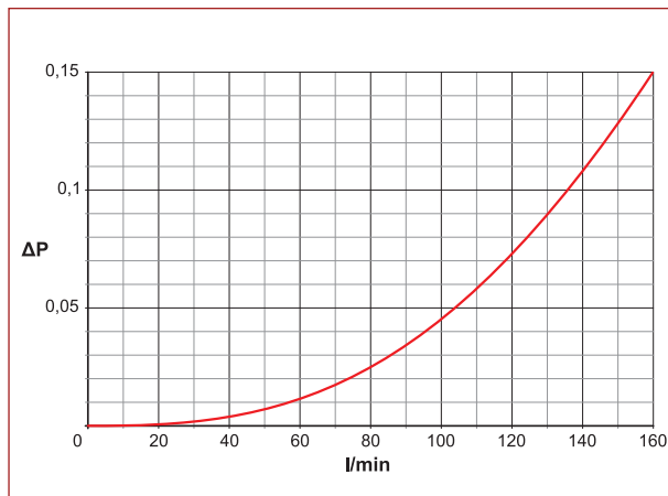
B con valvola with valve con válvula
